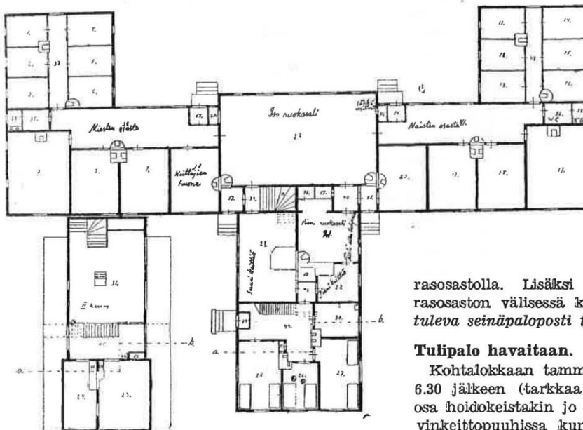
Pohjapiirros palaneesta kunnalliskodista. Palo alkoi pienestä ruokasalista (n:o 21). — Yllä kunnalliskoti ennen paloa.
